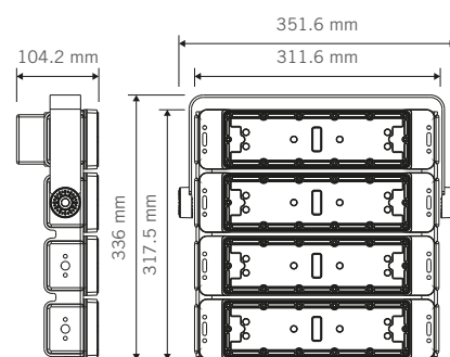
720301 - Modelo 200W
