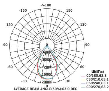
720300 - Modelo 150W
