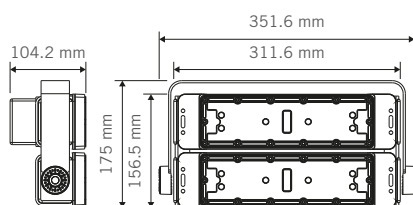
720299 - Modelo 100W
