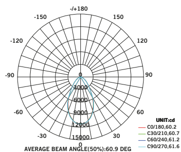
720299 - Modelo 100W
