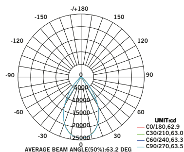
720301 - Modelo 200W
