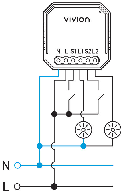
Diagrama de cableado
